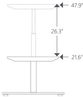
2-Leg Modular Frames [CGSAMOD-2LS & CGSAMOD-2L] Height Range
